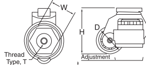
Stud Mount
